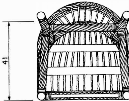
VISTA INFERIOR
