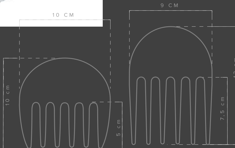
PLANOS GENERALES - PEINES EN MADERA
