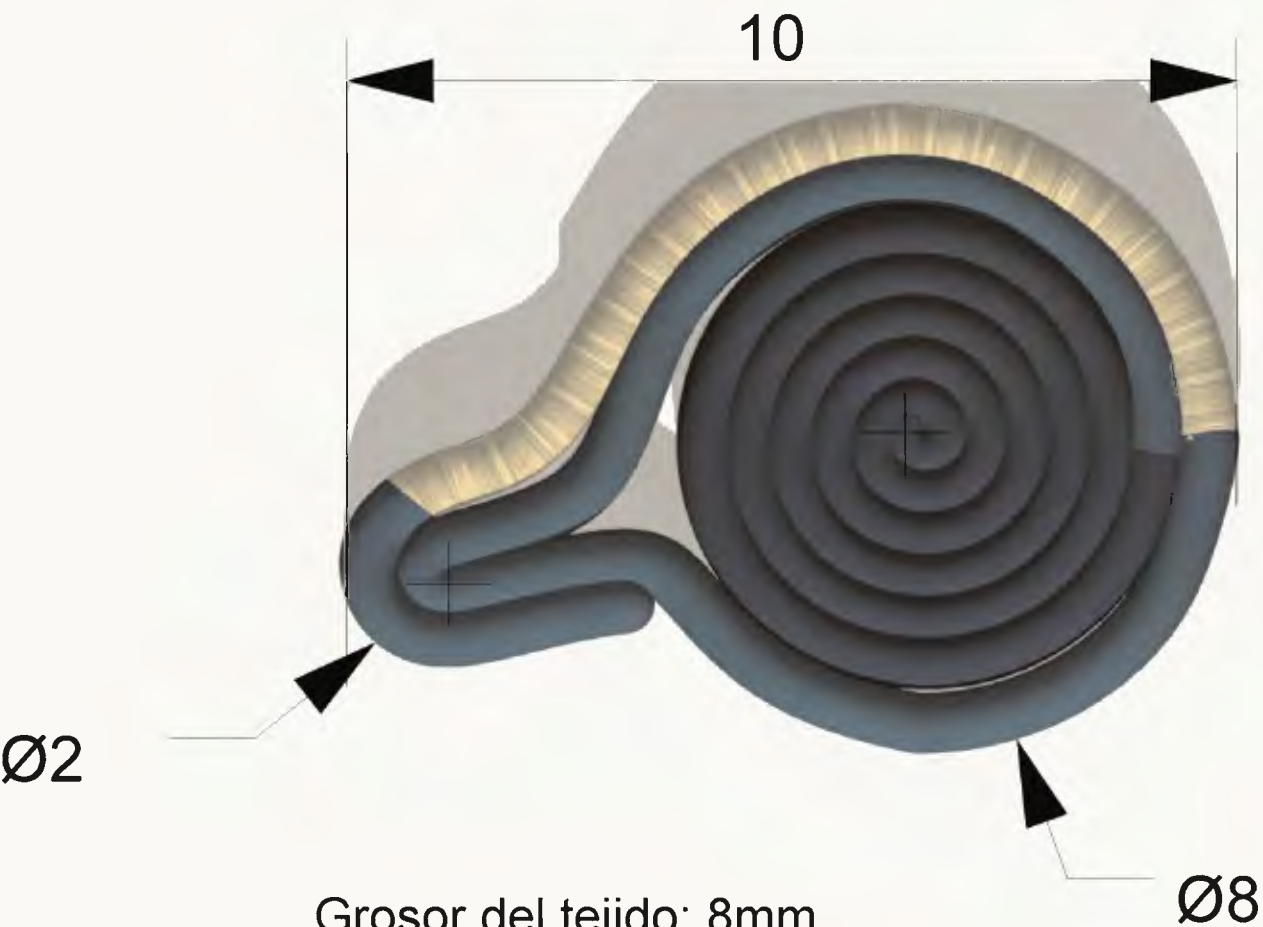
Vista Superior
