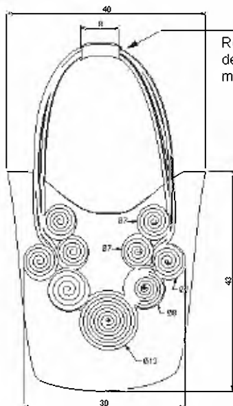
Vista Superior
