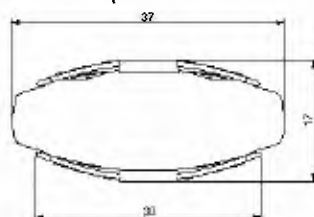
Vista Superior
